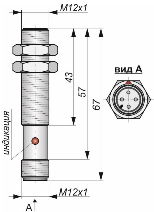
Габаритный чертеж
