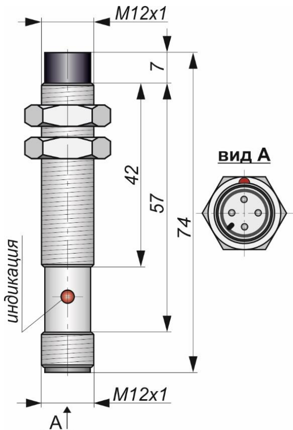
Габаритный чертеж
