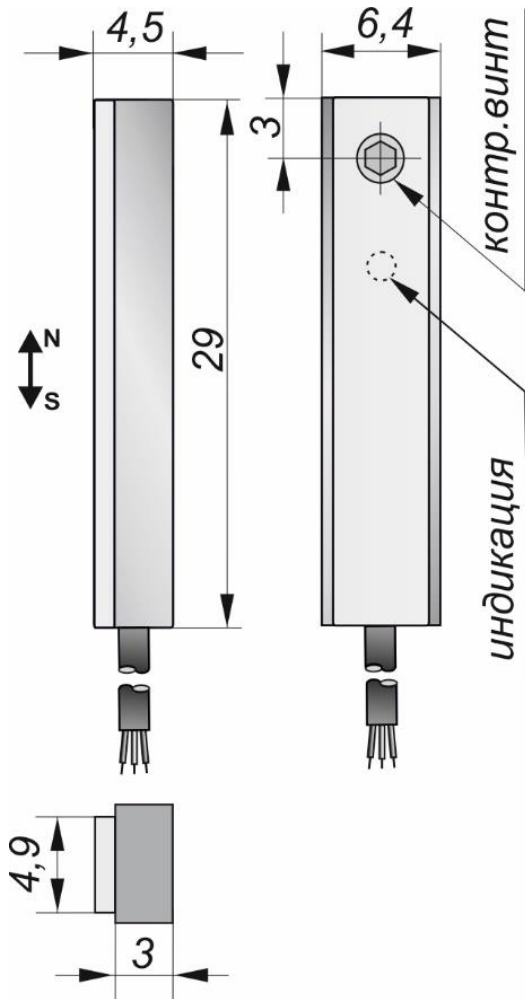
Габаритный чертеж
