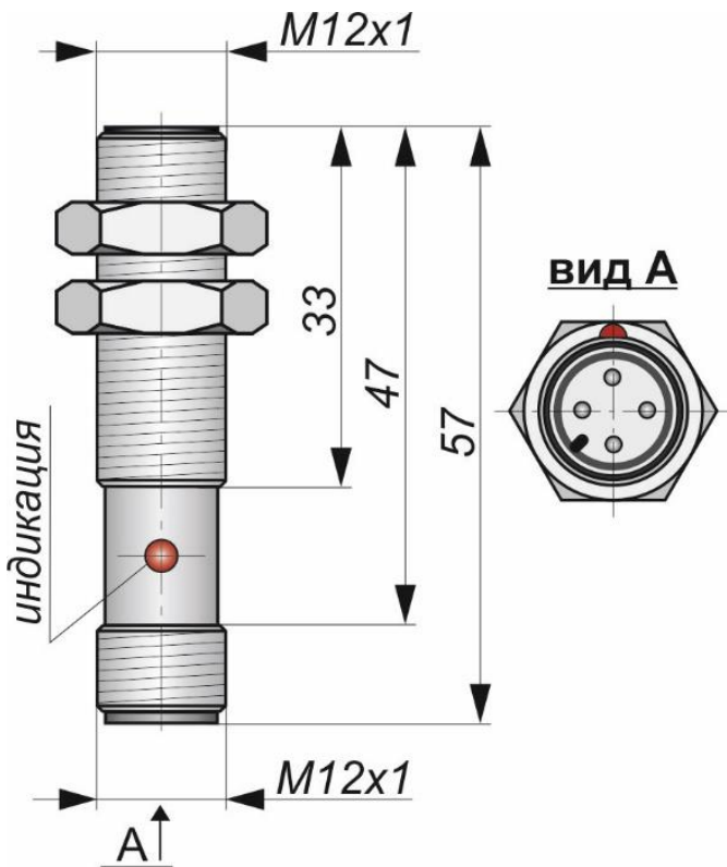
Габаритный чертеж
