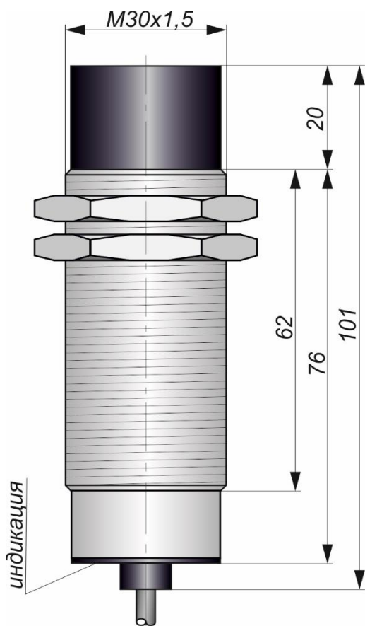
Габаритный чертеж
