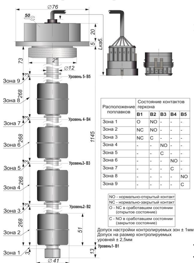
Габаритный чертеж
